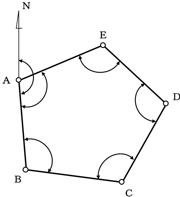
測点の概略図例
